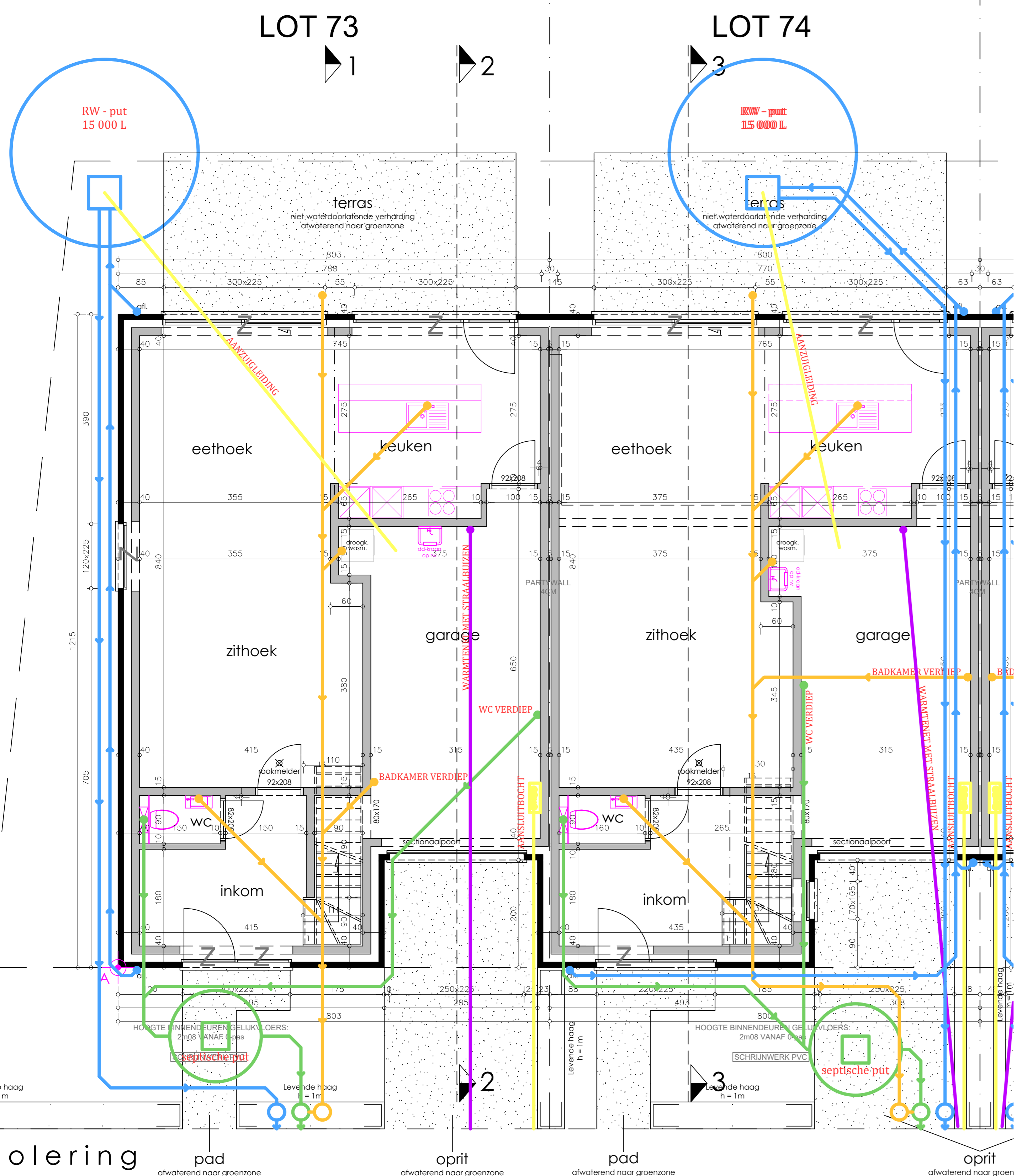
Gelijkvloers
