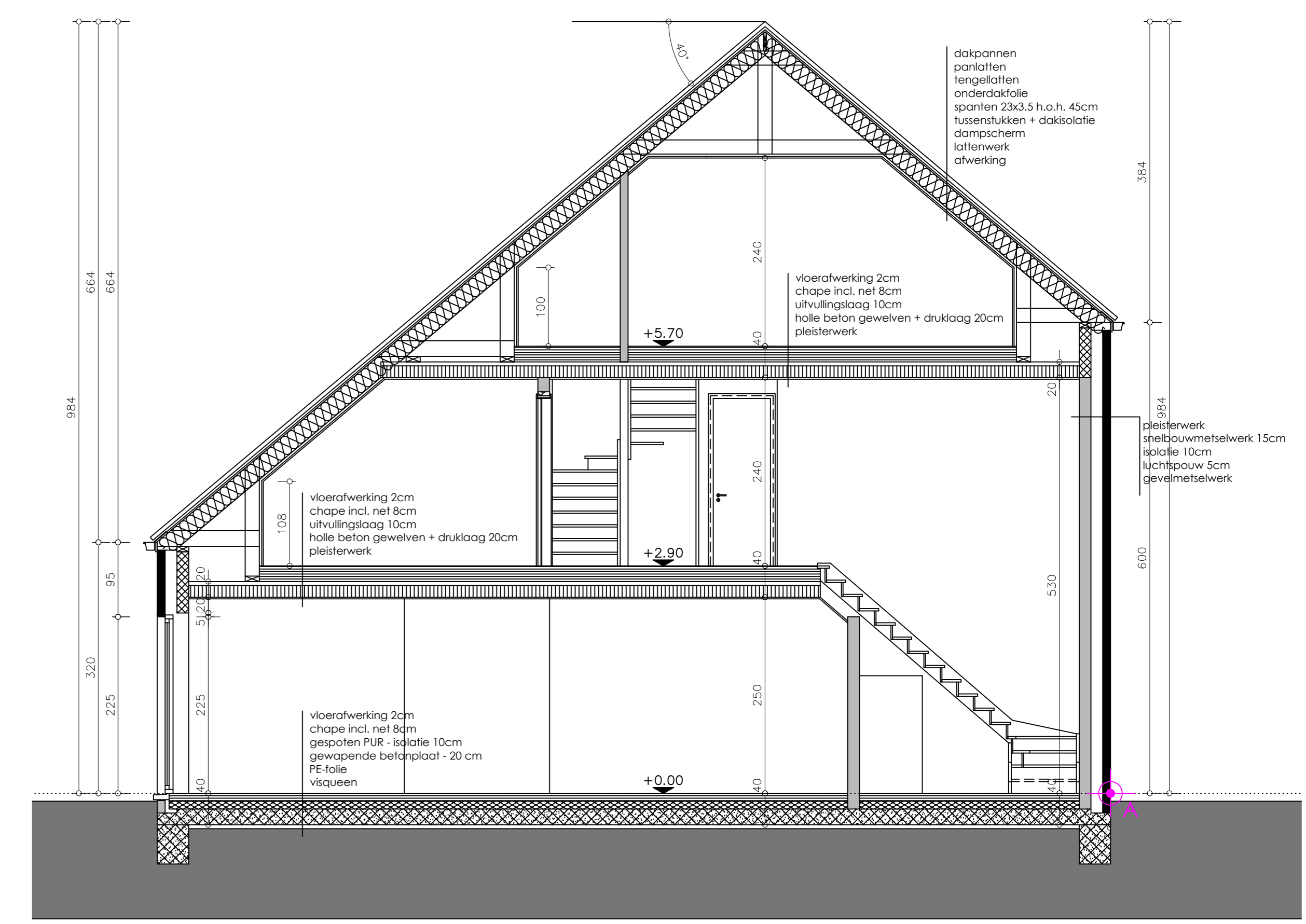
Doorsnede 1-1 (lot 73)
