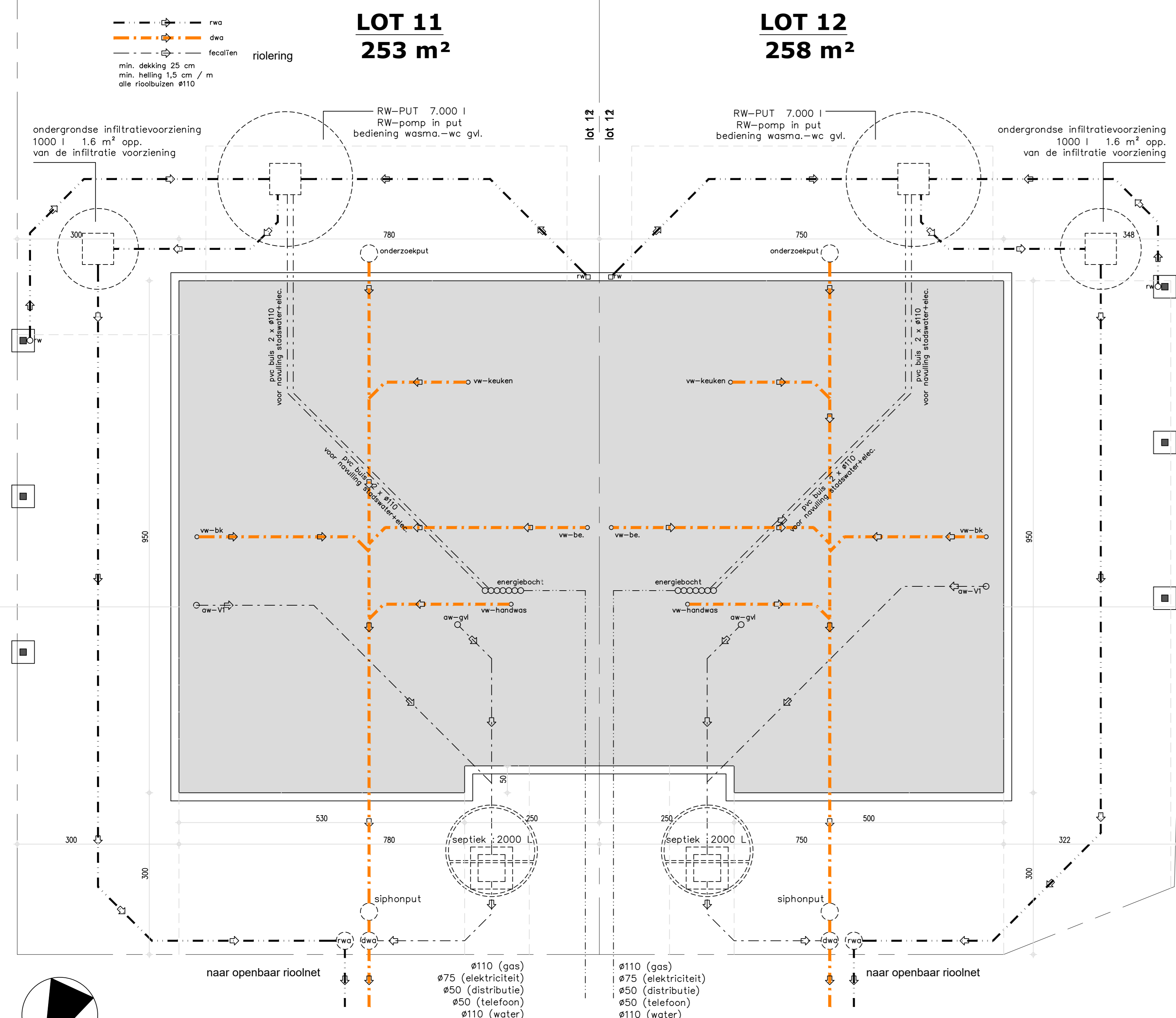
ONDERGROND - RIOLERING 1/50
