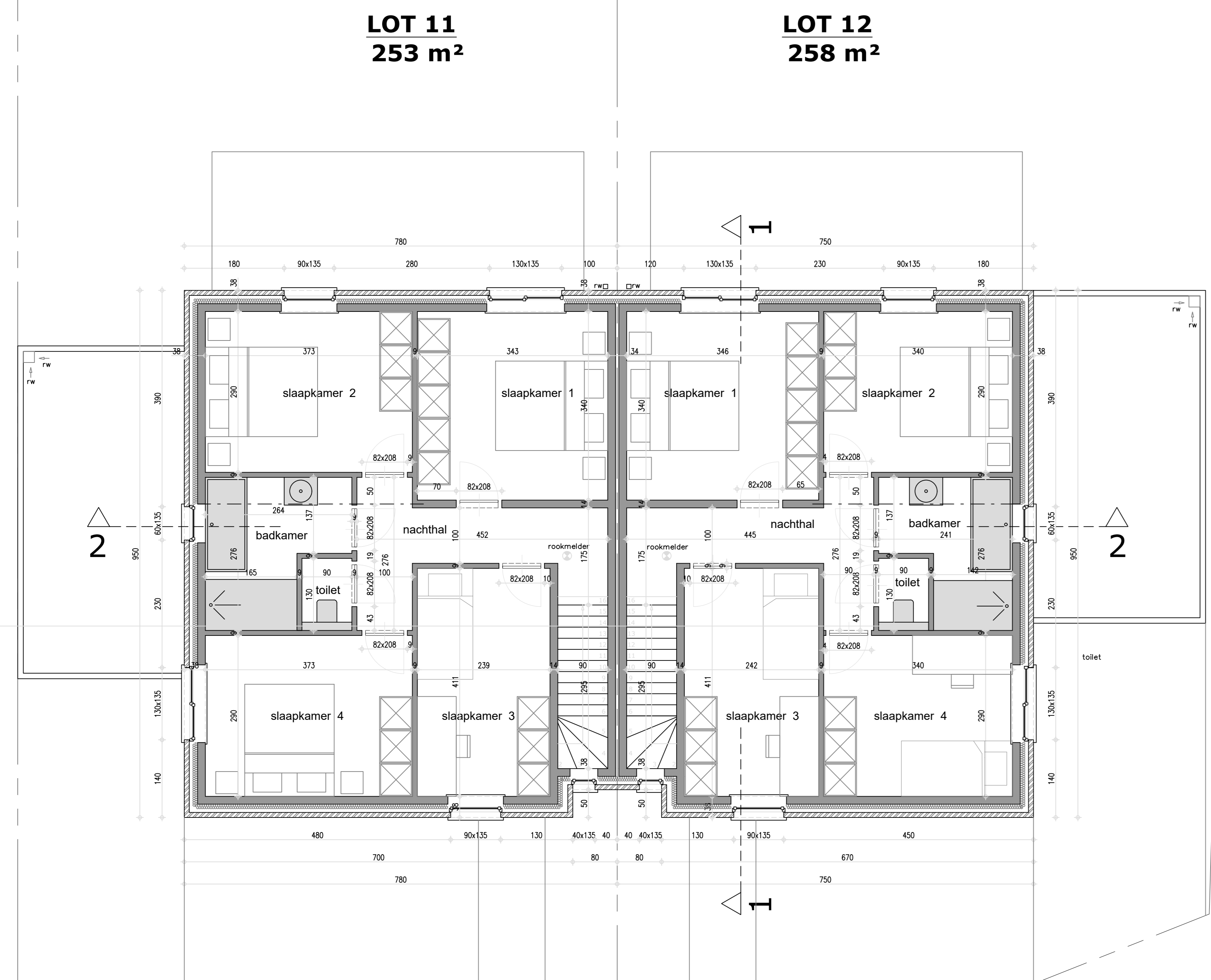
VERDIEPING 1 1/50
