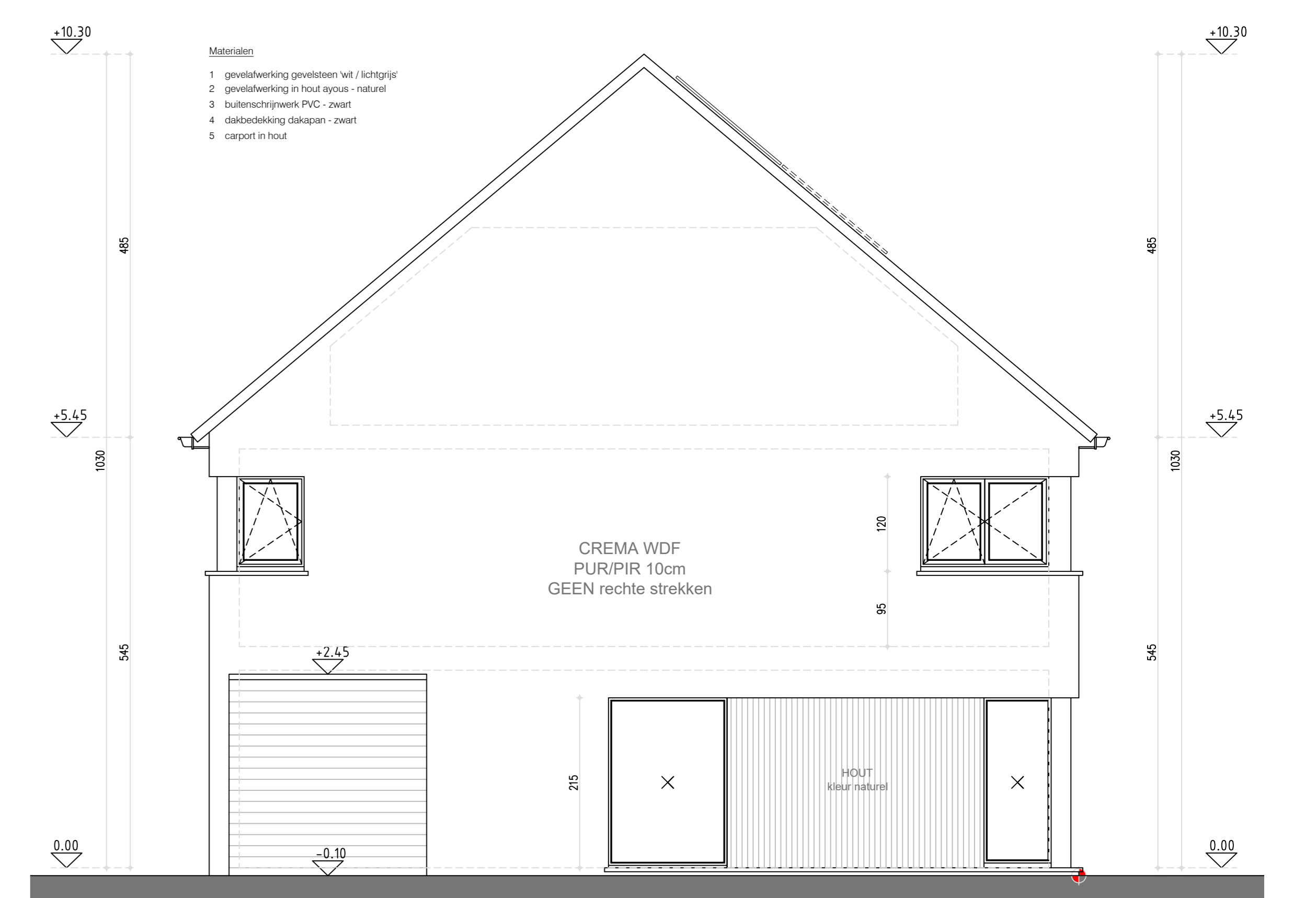
gevel west - rechter zijgevel lot 3
