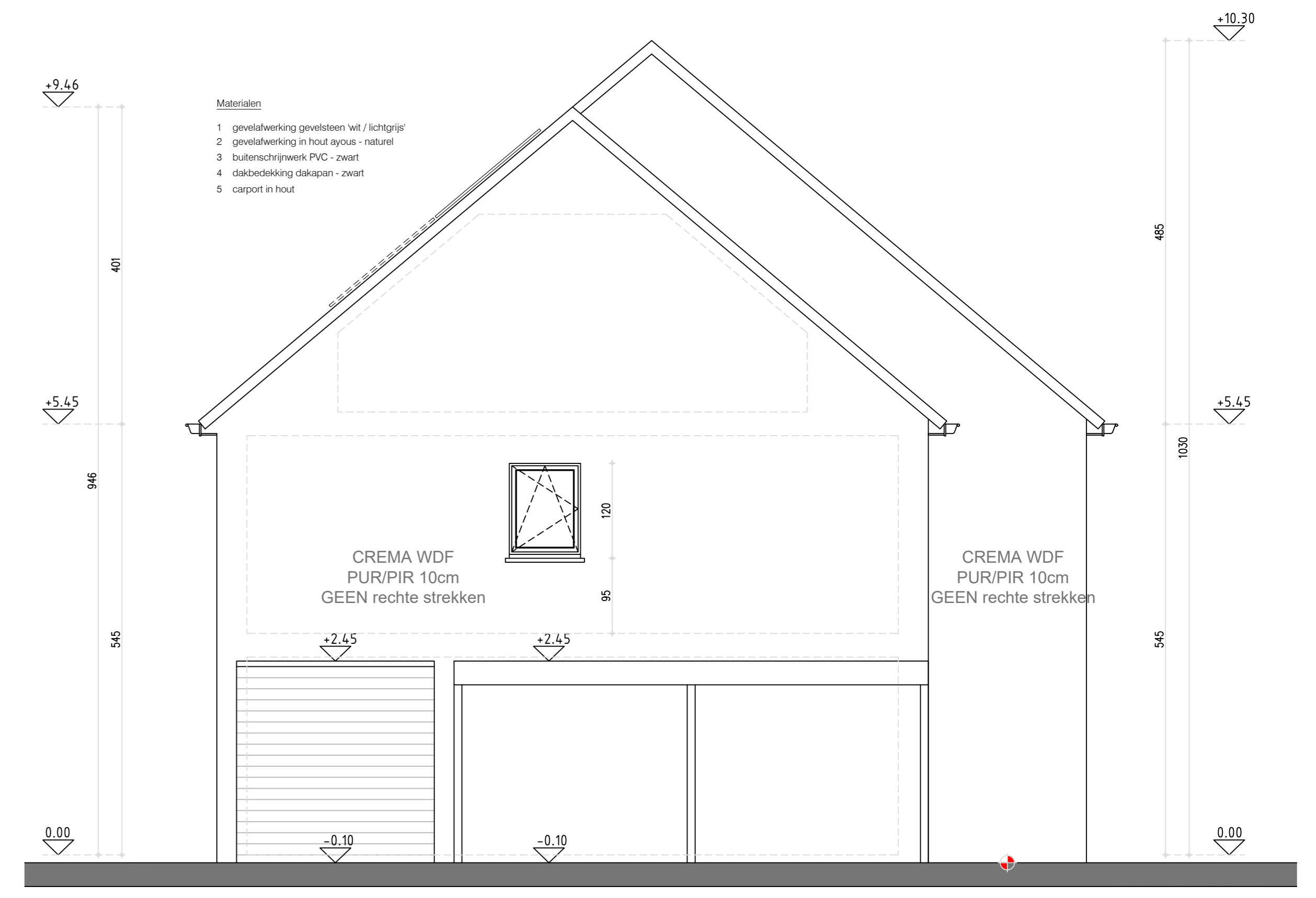
gevel oost - linker zijgevel lot 4
