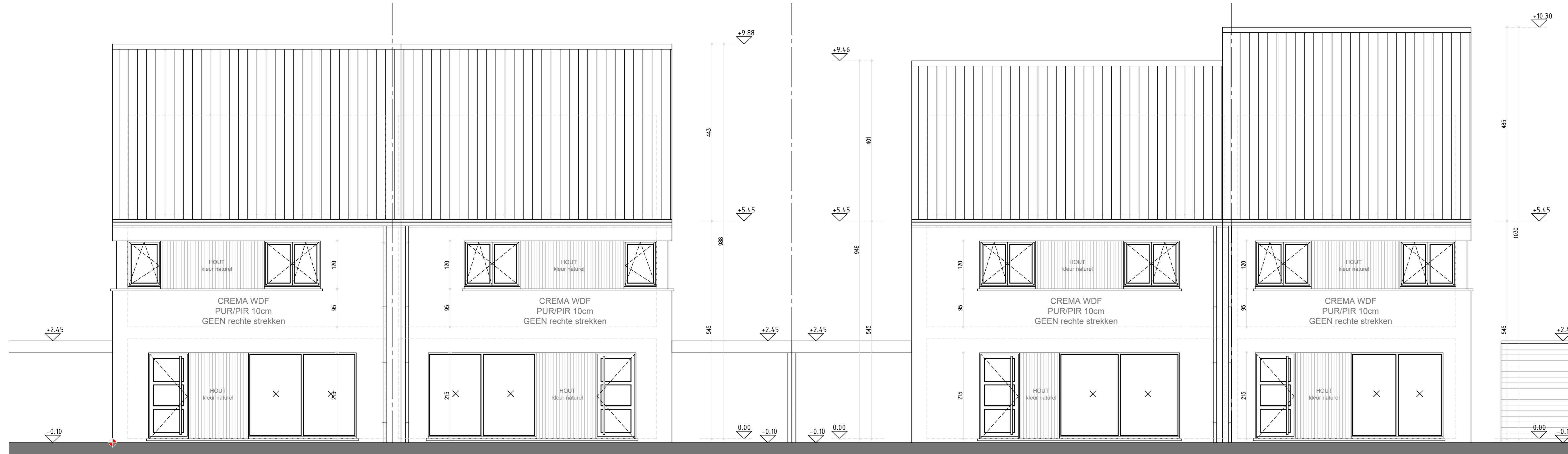
gevel noord - voorgevel lot 6
