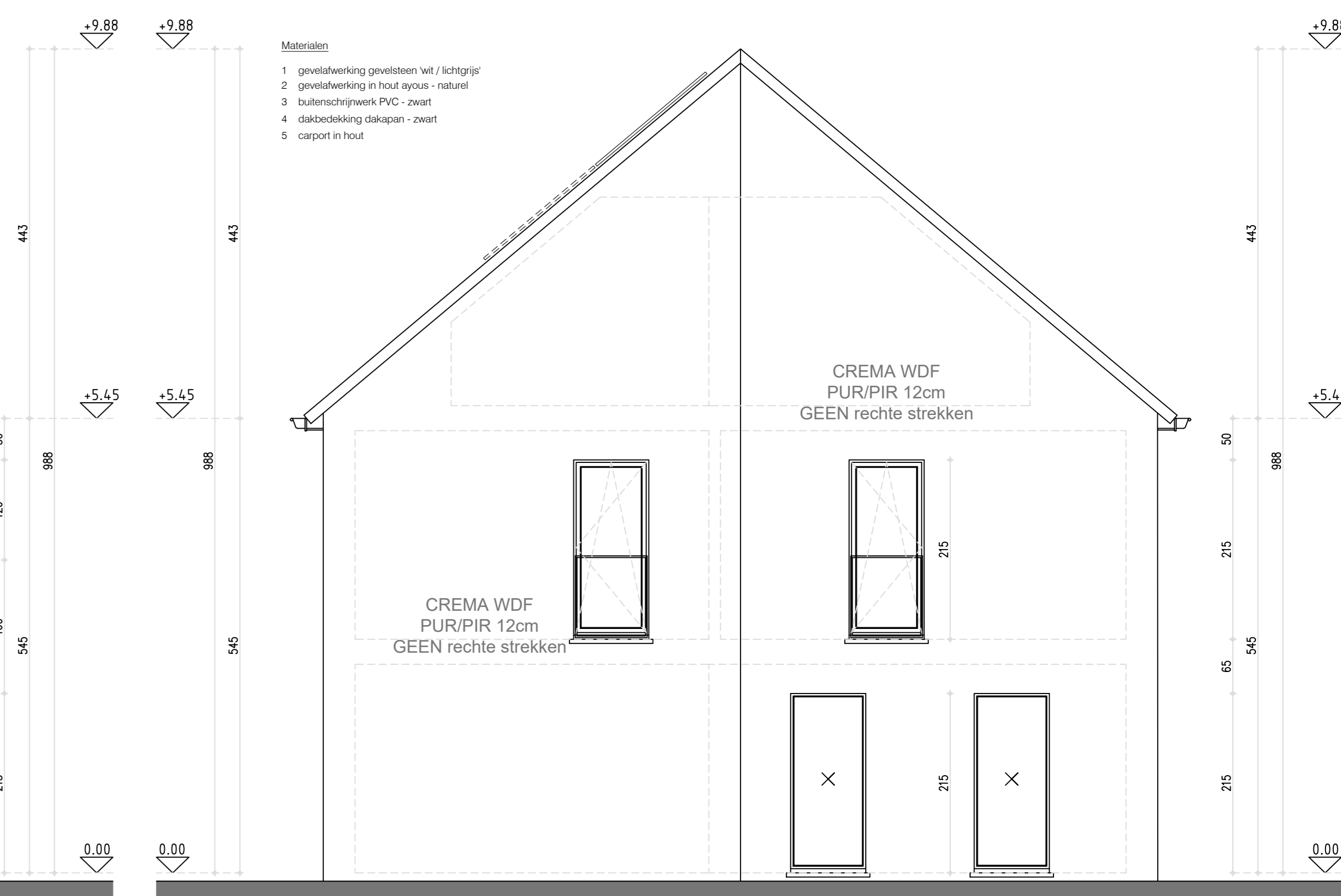
gevel oost - linker zijgevel lot 7
