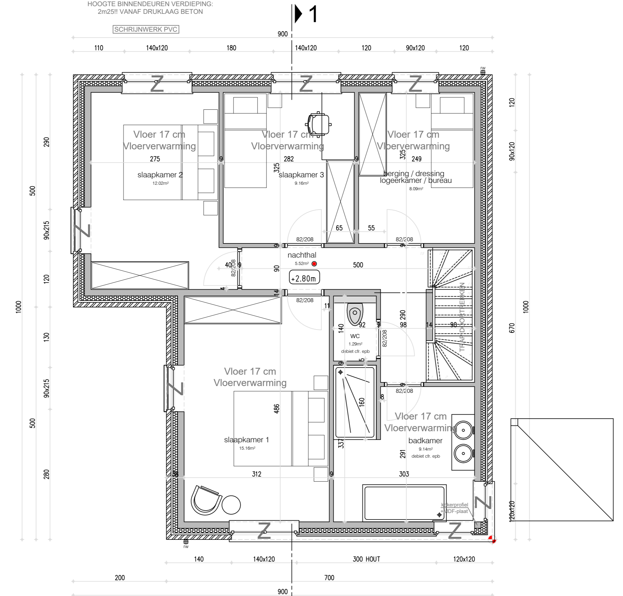
verdiepingsplan lot 7 80.00 m² bruto opp. 66.13 m² netto opp.
