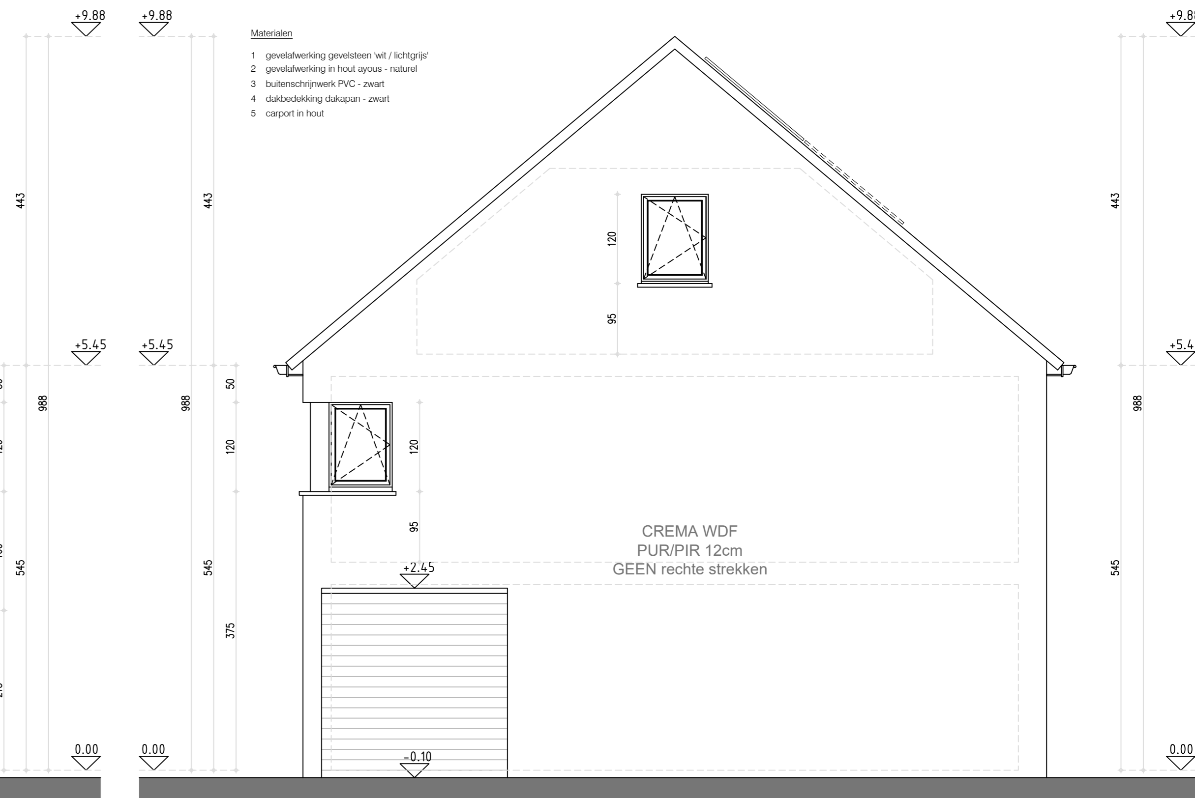
gevel west - rechter zijgevel lot 7
