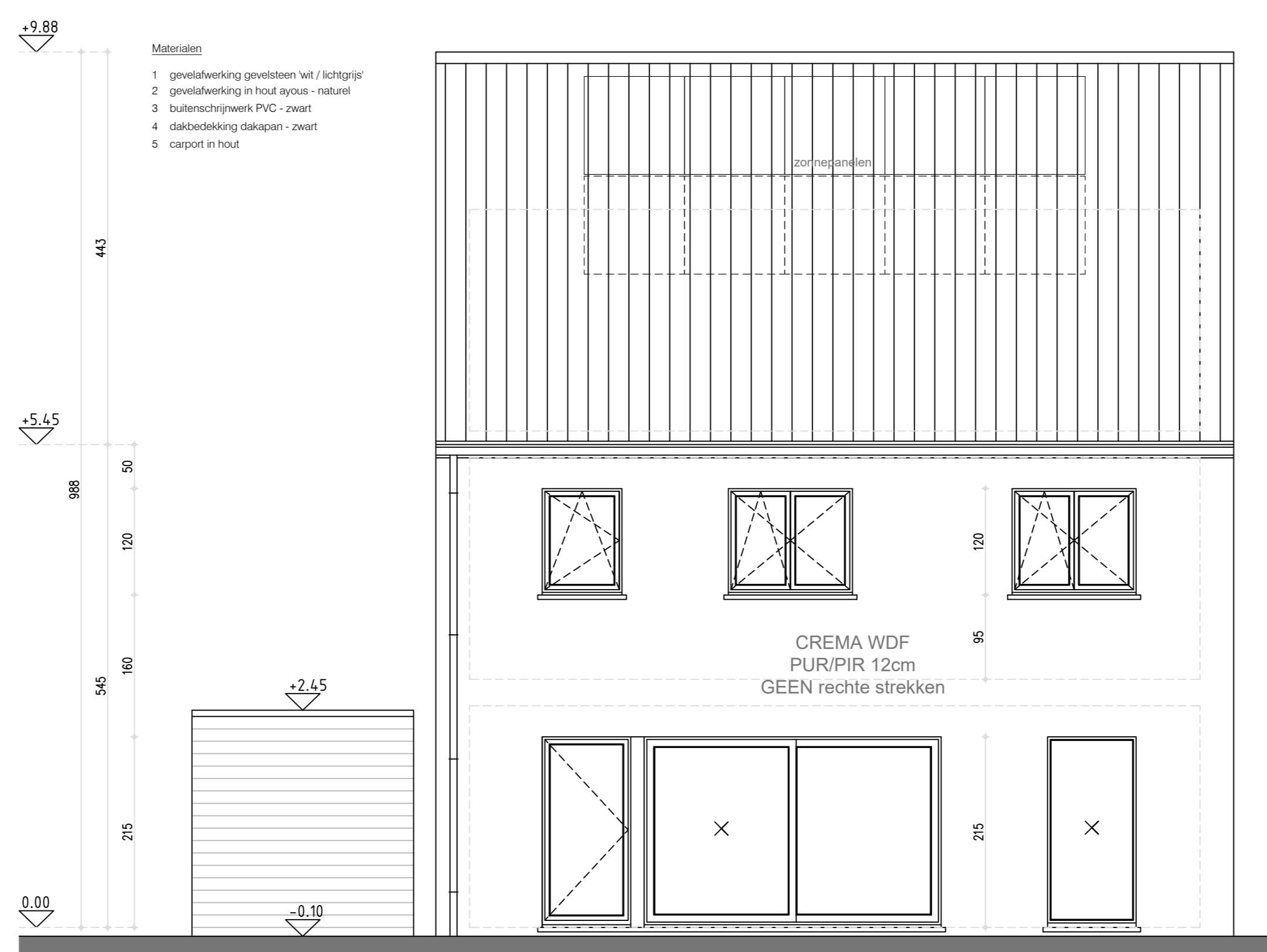
gevel zuid - achtergevel lot 7
