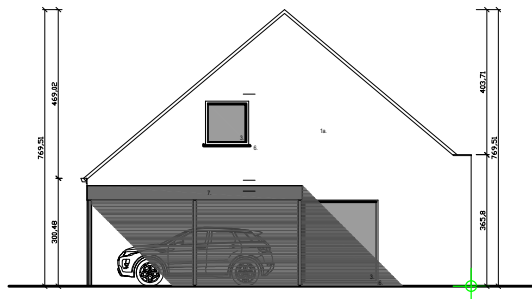
WONING 2 Zijgevel Links
