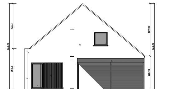
WONING 3 Zijgevel Rechts
