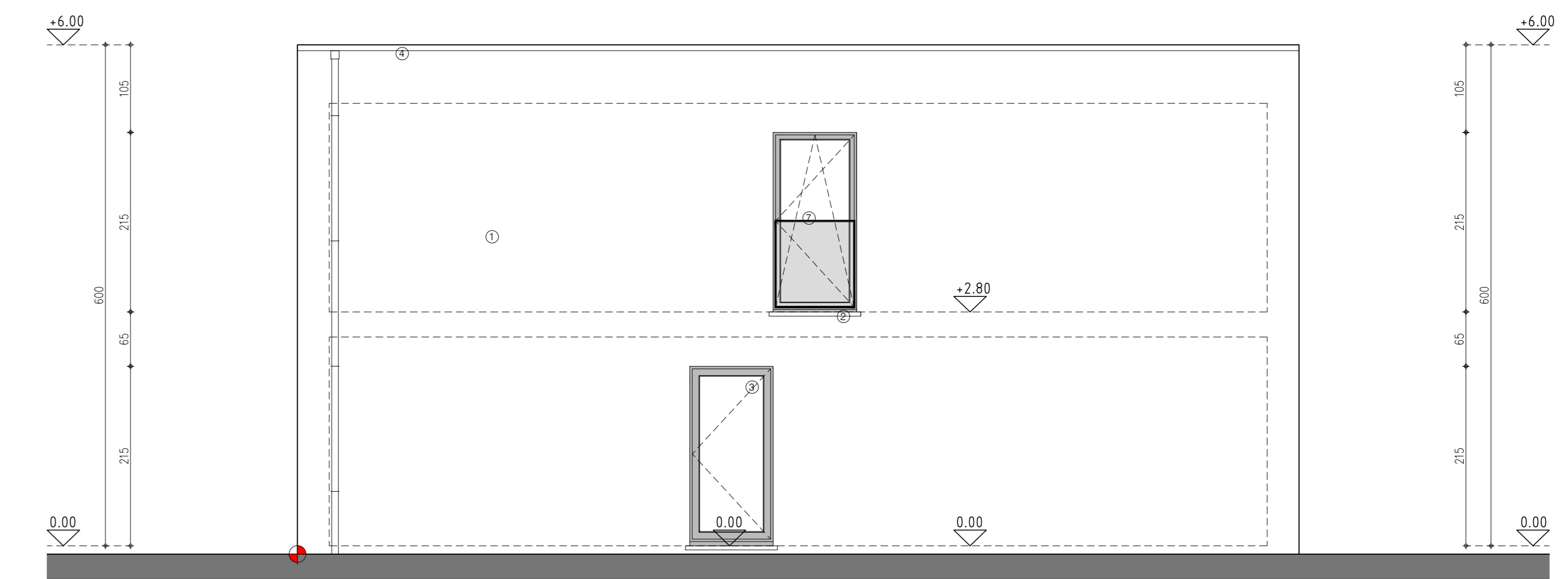
gevel oost - rechter zijgevel lot 78
