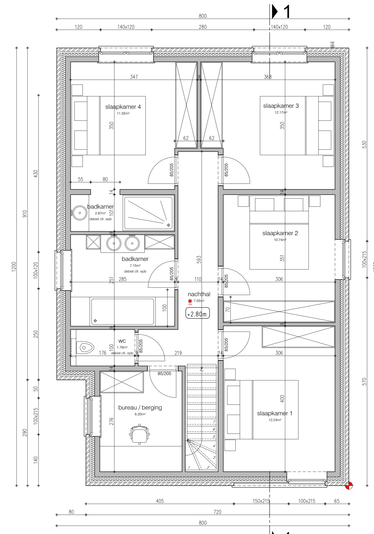
verdiepingsplan lot 78 93.68 m 2 bruto opp. 79.05 m 2 netto opp.
