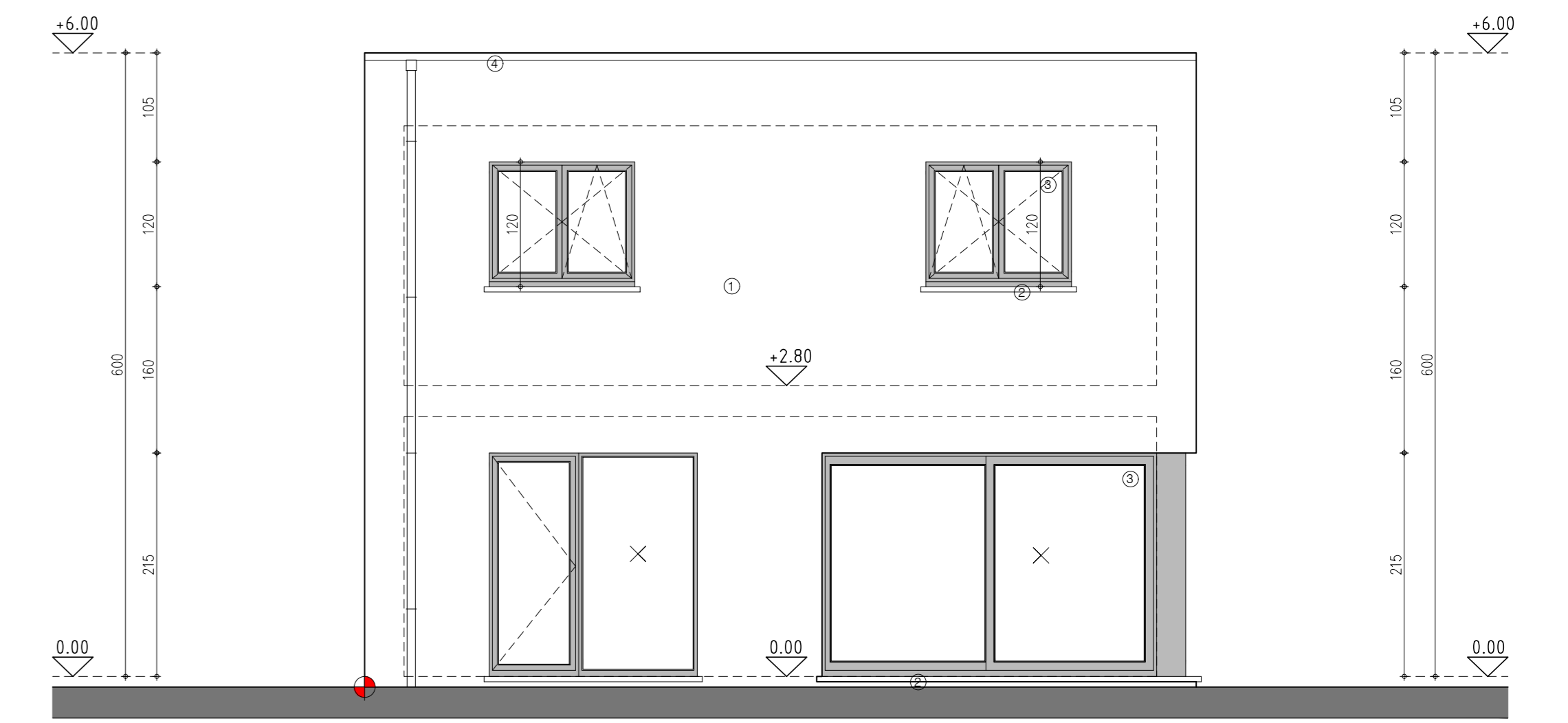
gevel noord - achtergevel lot 78
