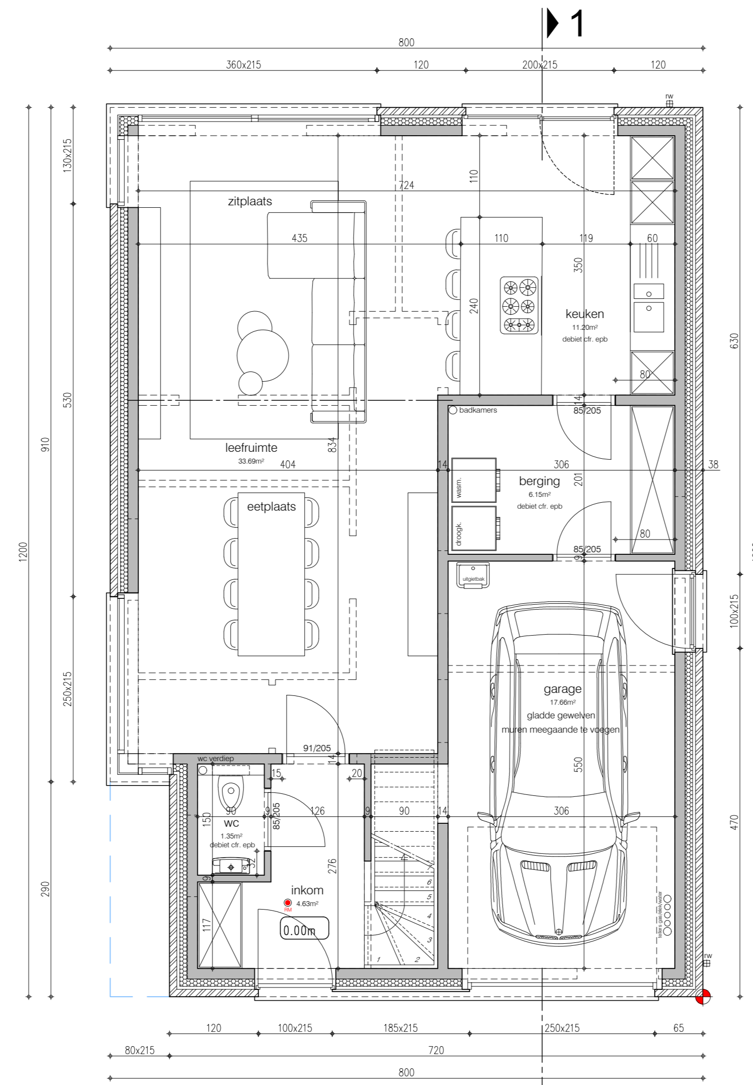
gelijkvloers lot 78 93.68 m 2 bruto opp. 79.05 m 2 netto opp.
