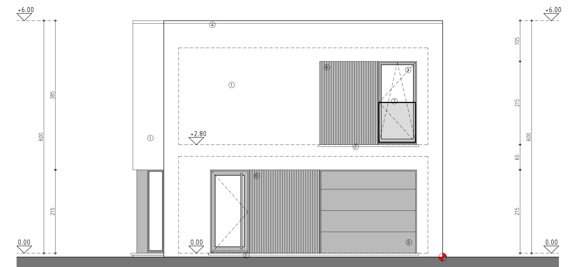
gevel zuid - voorgevel lot 78
