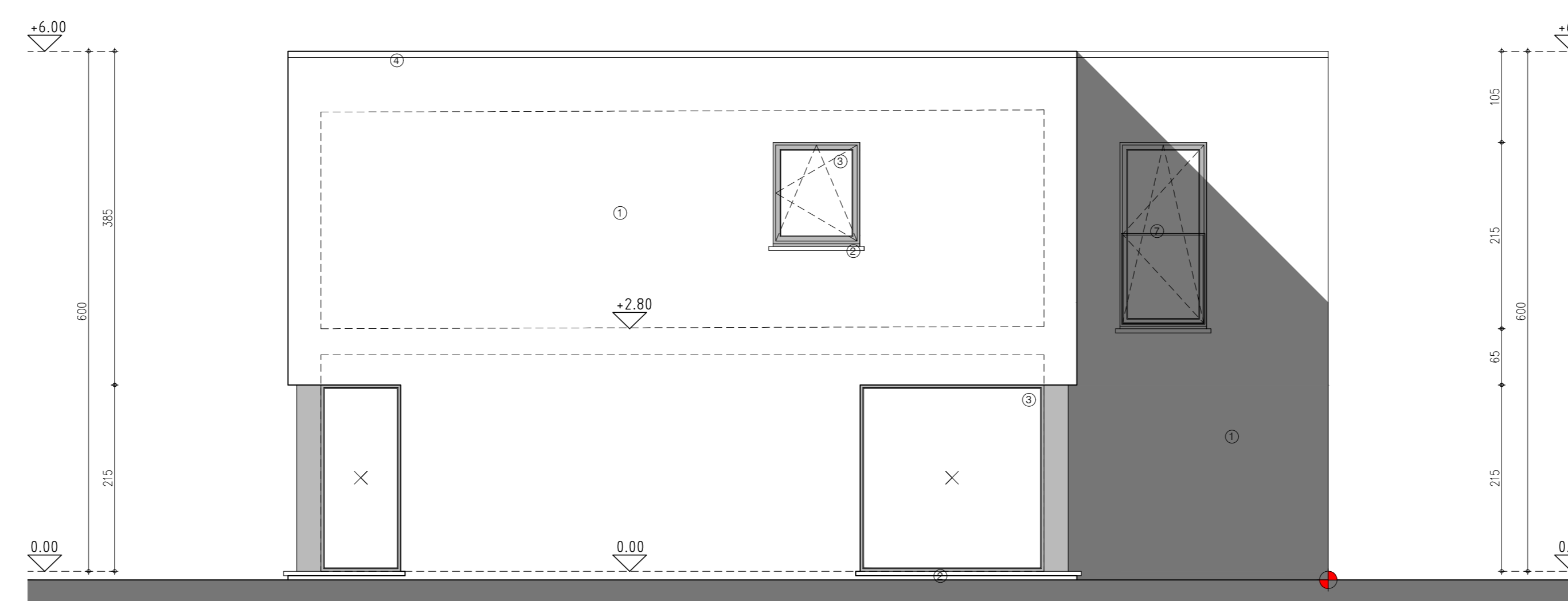
gevel west - linker zijgevel lot 78
