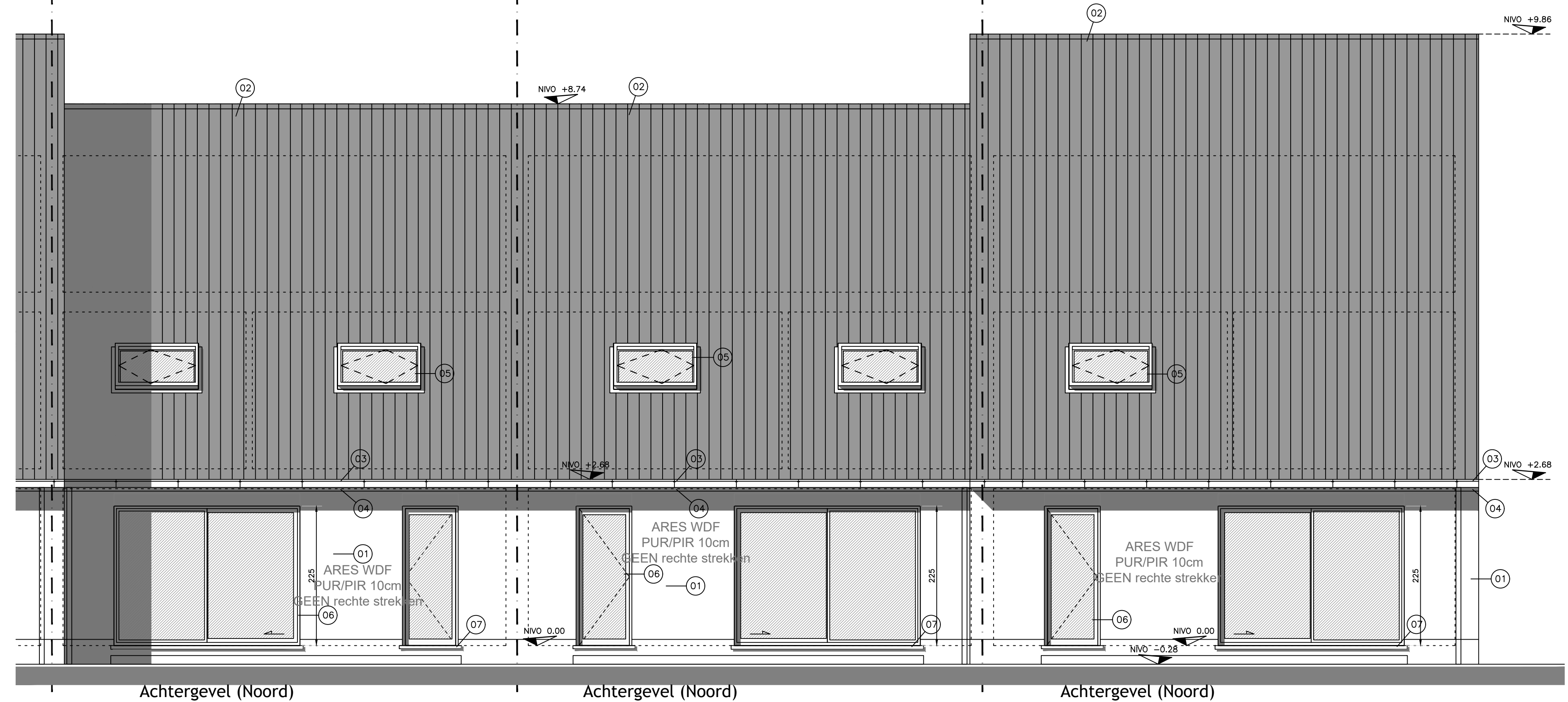
Achtergevel (Noord) Lot 14
