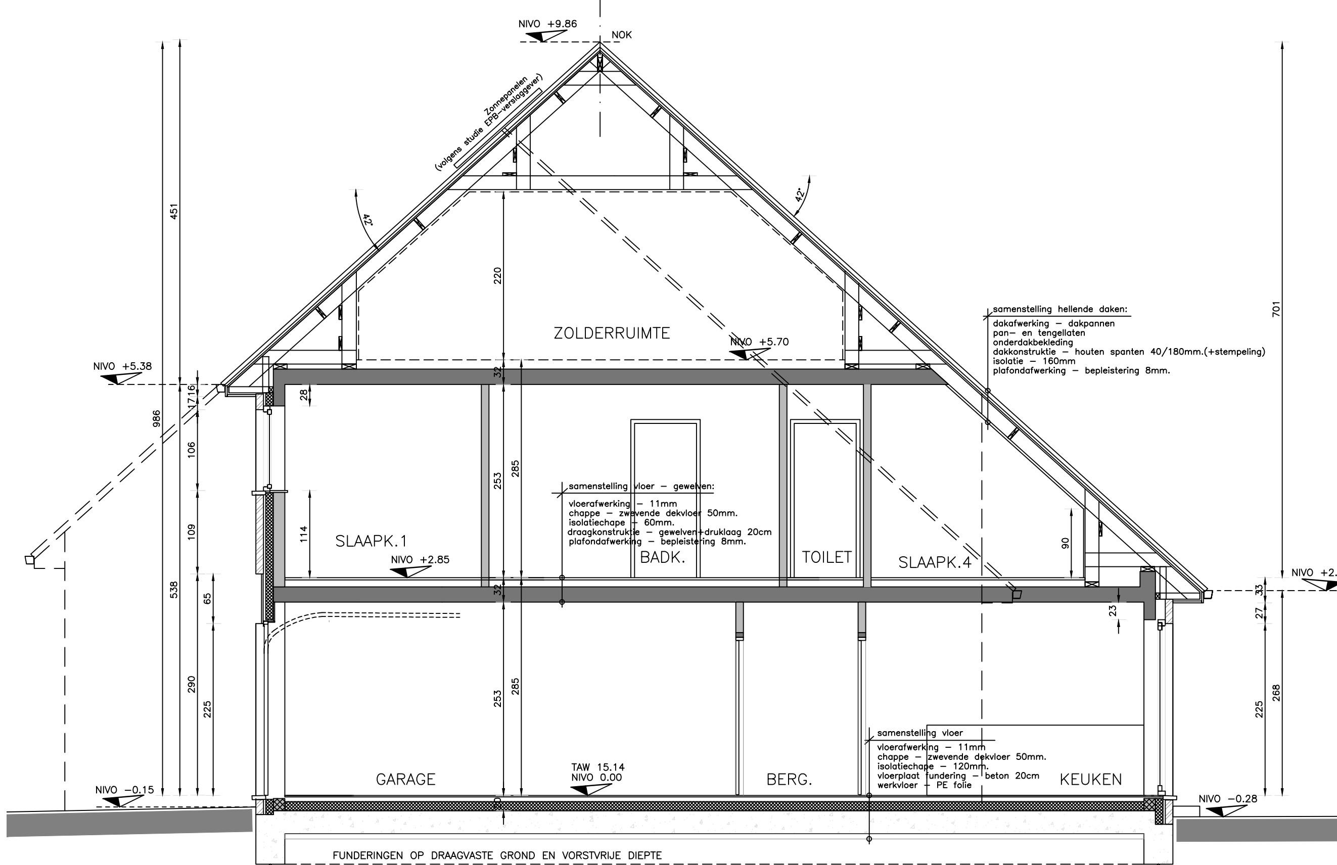
Doorsnede I-I Lot 16
