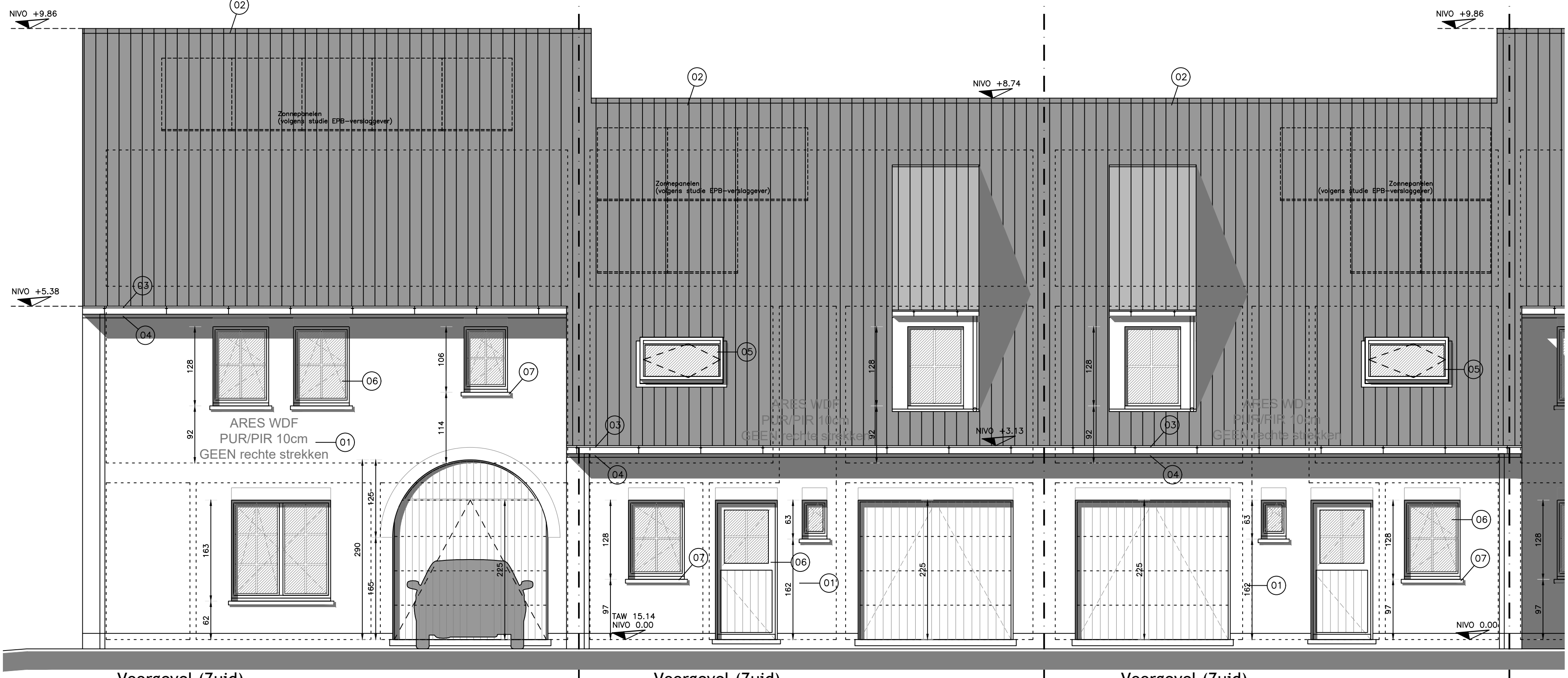
Voorgevel (Zuid) Lot 16
