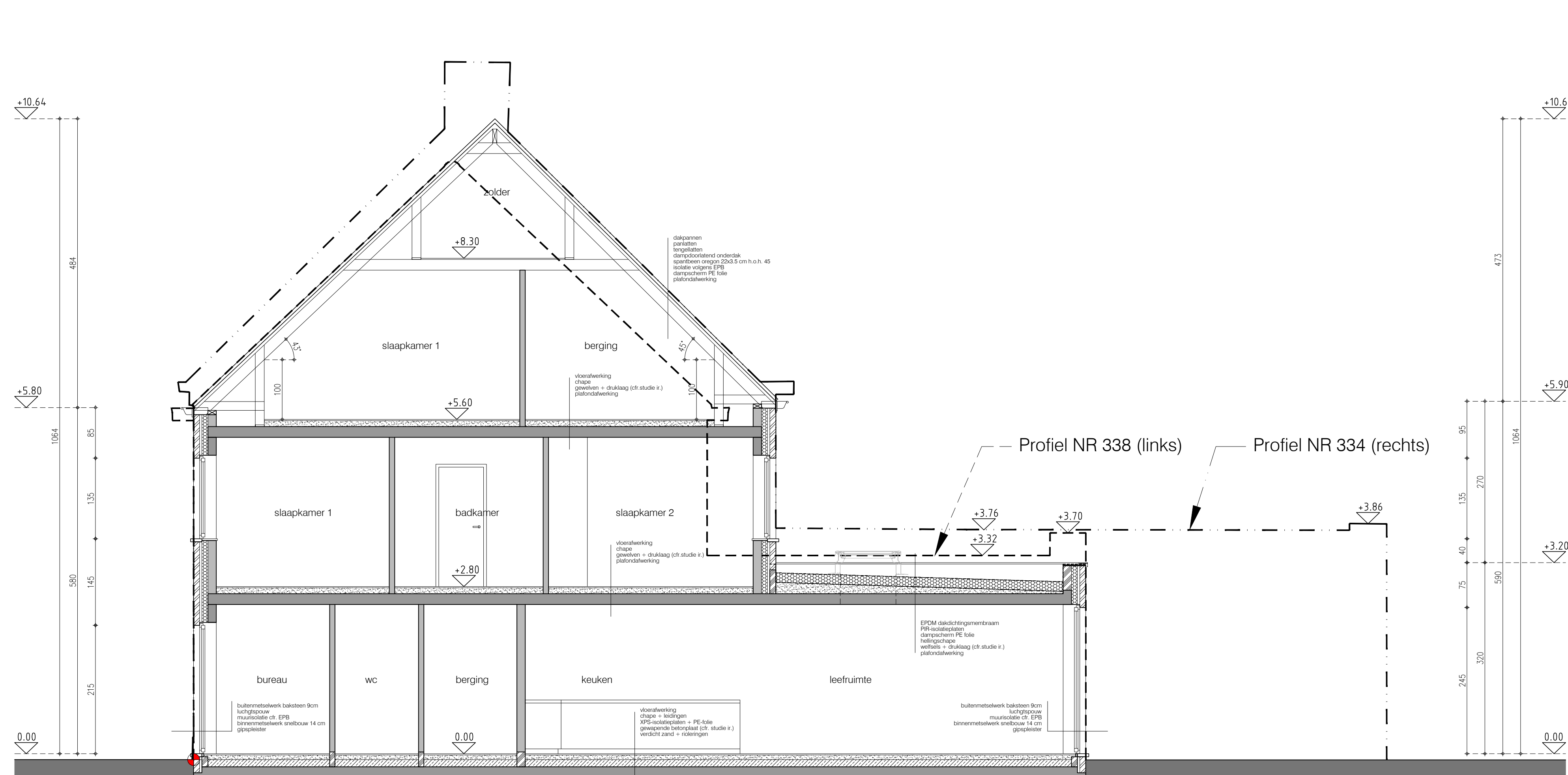
doorsnede 1-1
