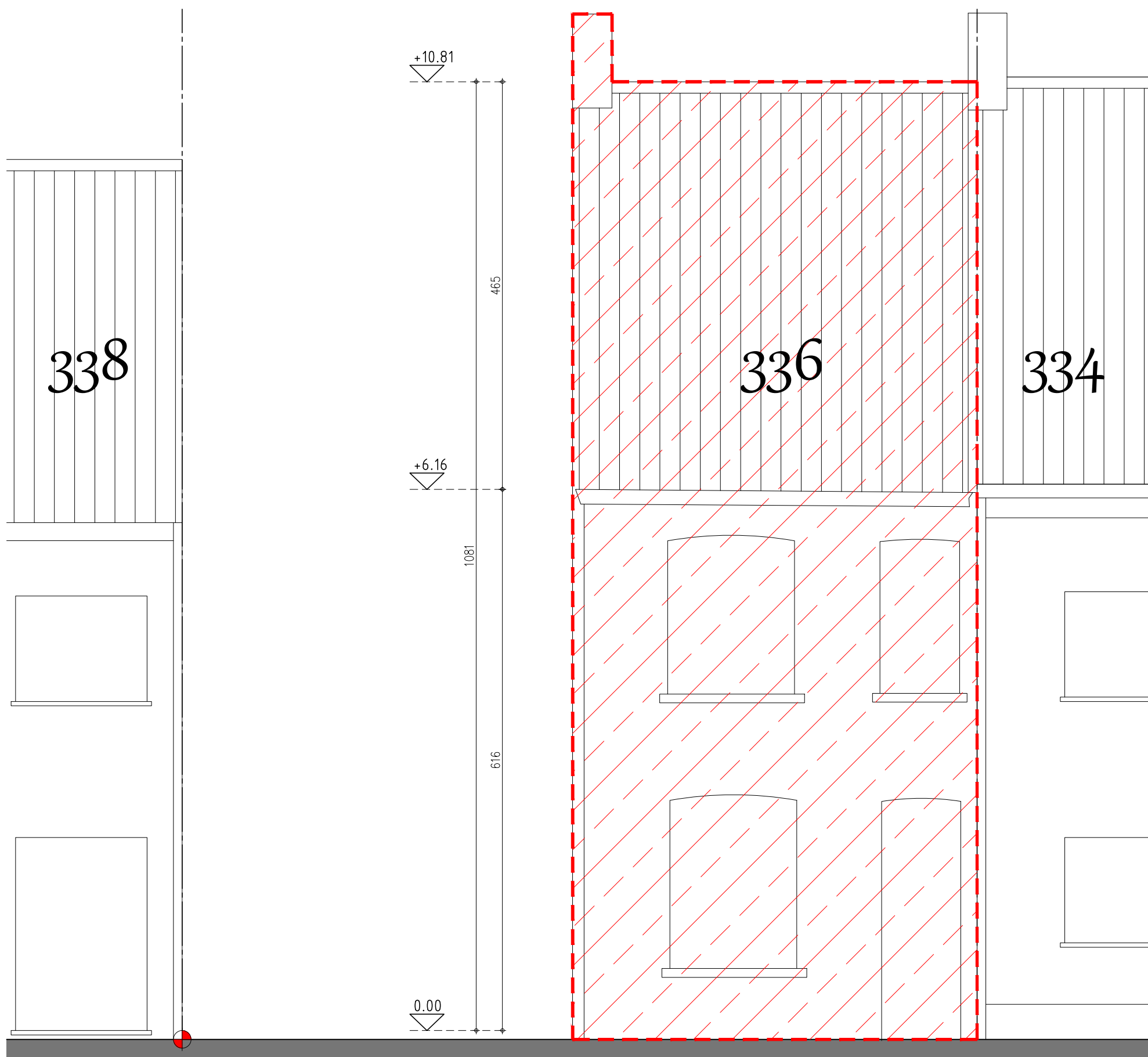
gevel oost - voorgevel - bestaande toestand TE SLOPEN WONING
