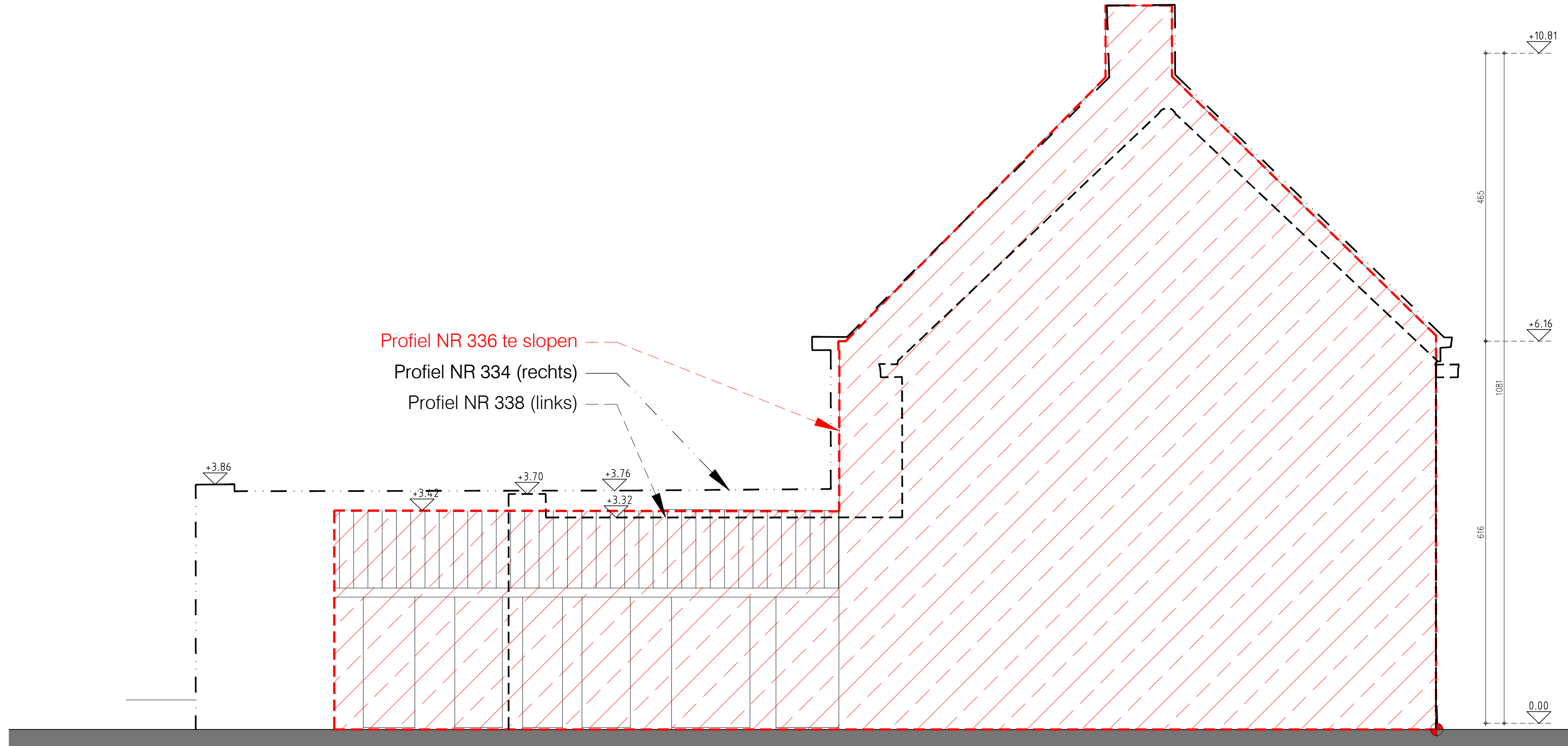
gevel zuid - zijgevel - bestaande toestand TE SLOPEN WONING
