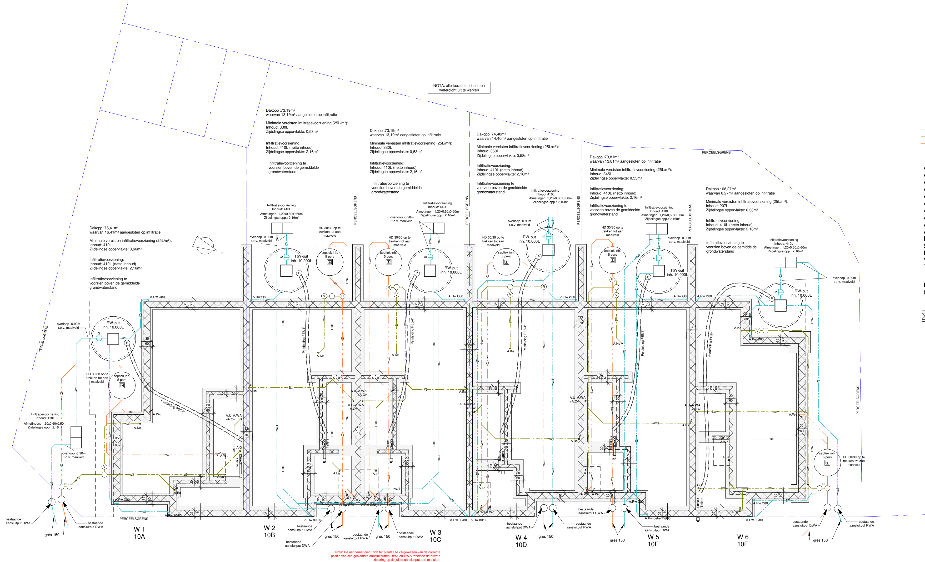
3 - 10 Funderings en Rioleringsplan 1 : 100
