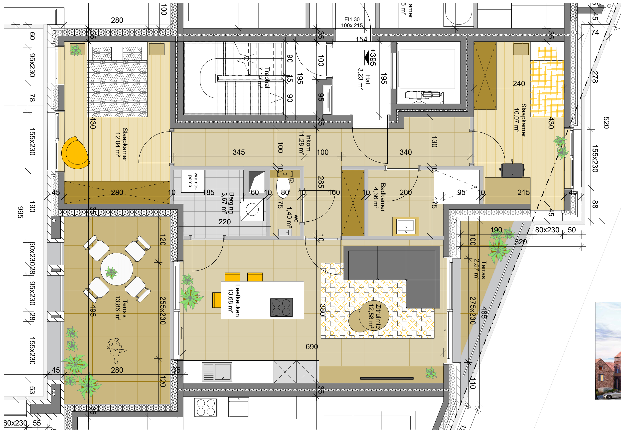
VERDIEPING 1 SCHAAL: 1/50
