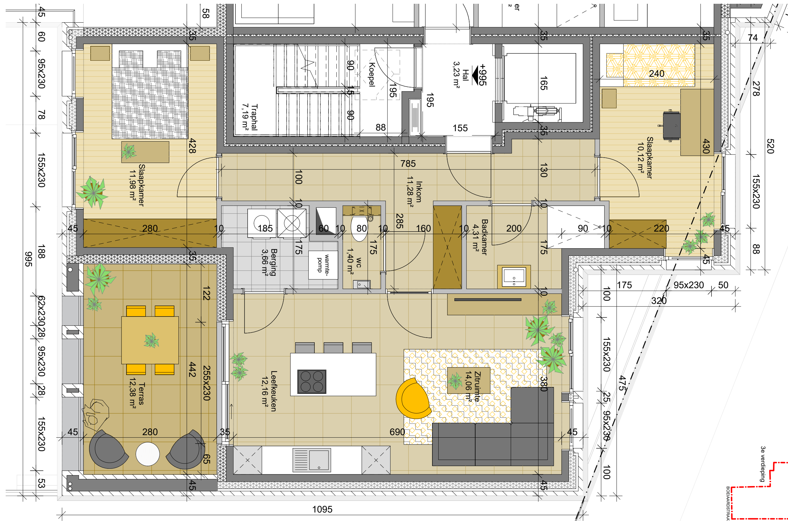
VERDIEPING 3 SCHAAL: 1/50
