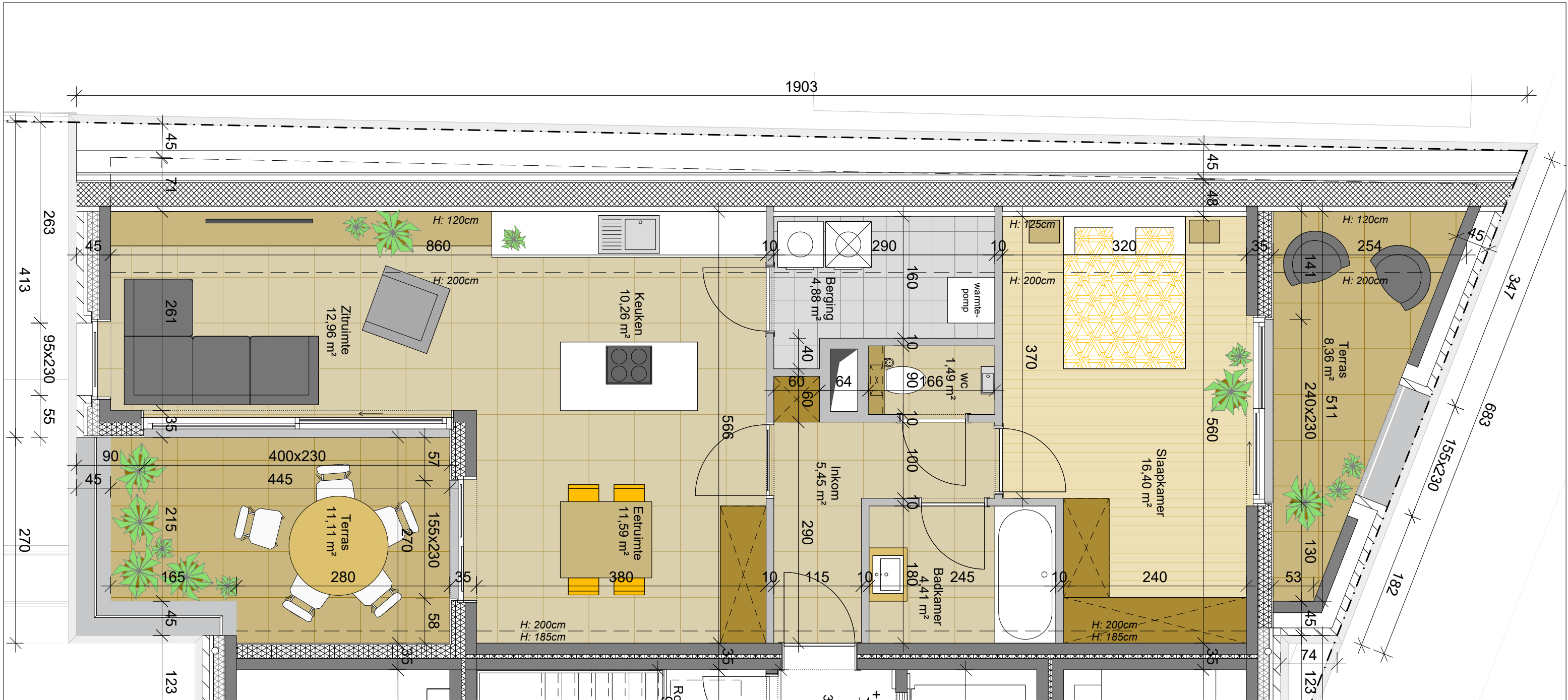
VERDIEPING 4 SCHAAL: 1/50
