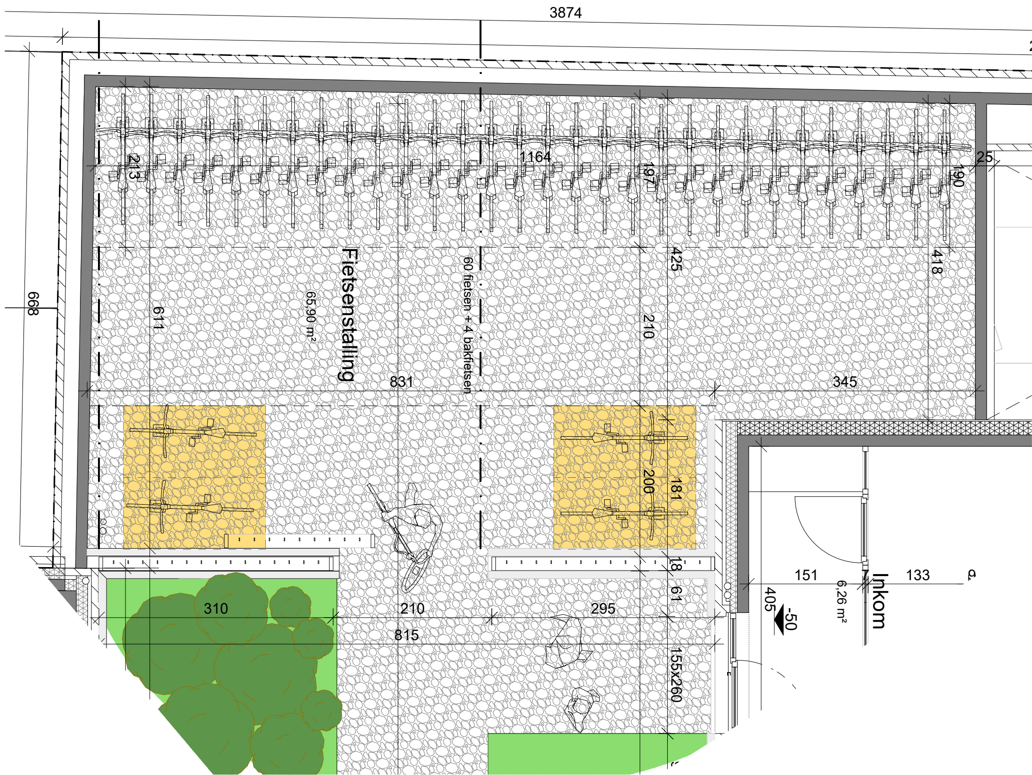
GELIJKVLOERS SCHAAL: 1/50
