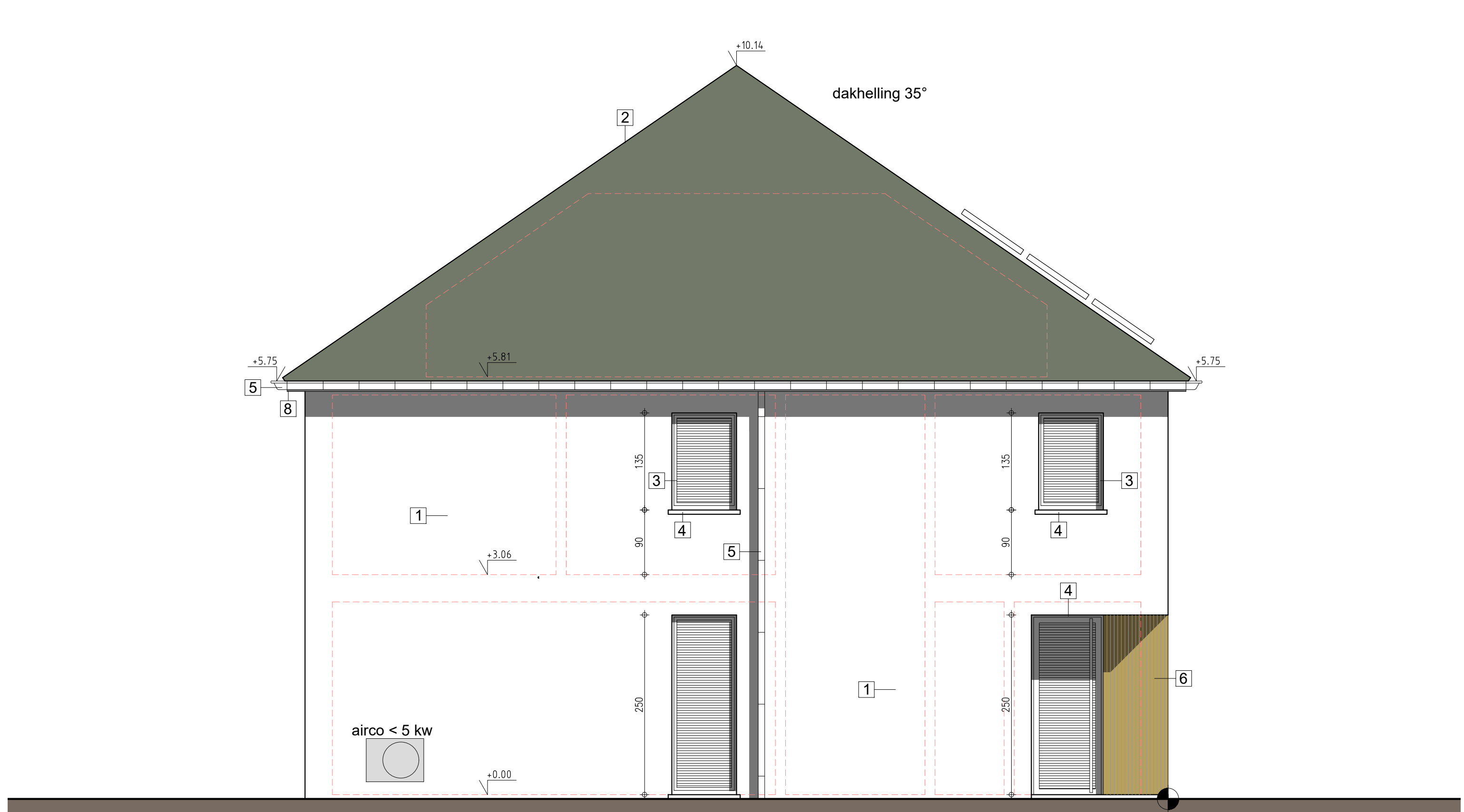
ZIJGEVEL LINKS : 1/50
