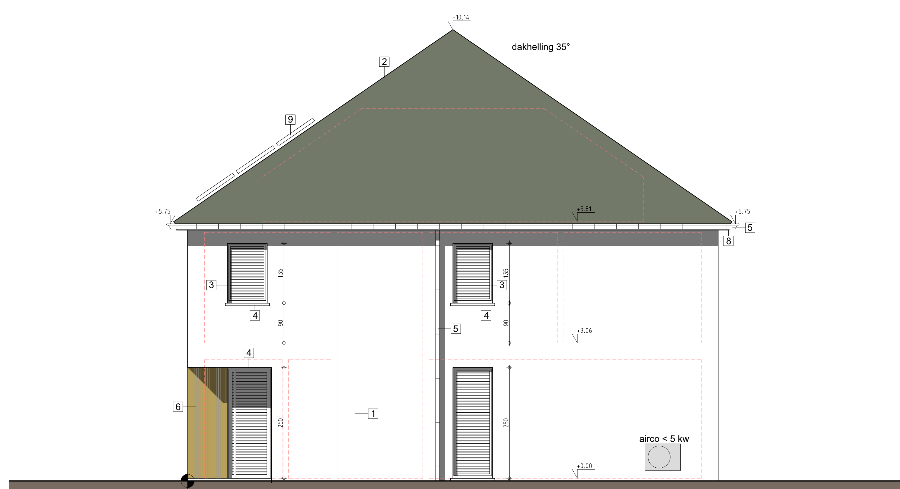
ZIJGEVEL RECHTS : 1/50
