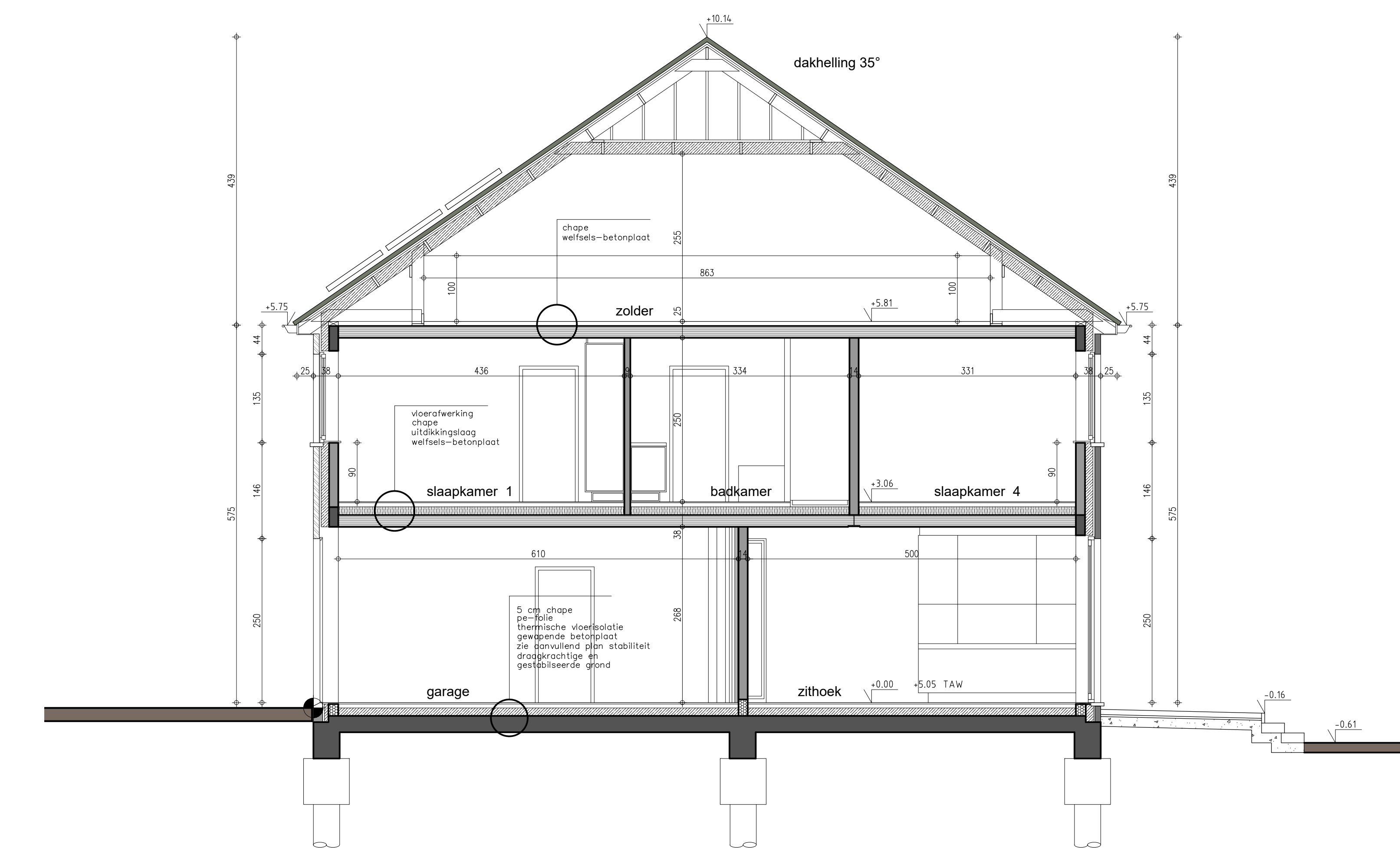
DOORSNEDE 1-1 : 1/50
