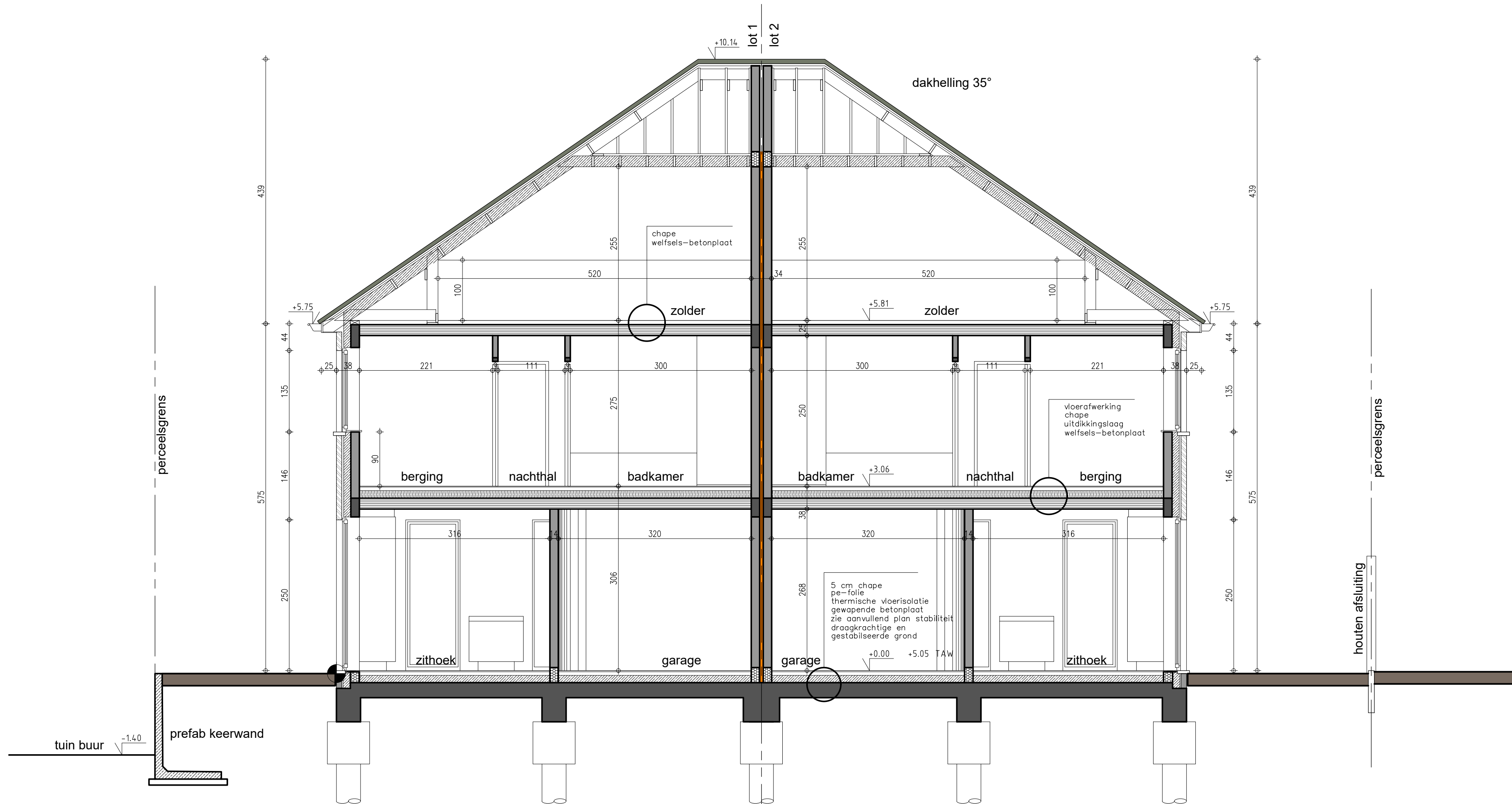
DOORSNEDE 2-2 : 1/50
