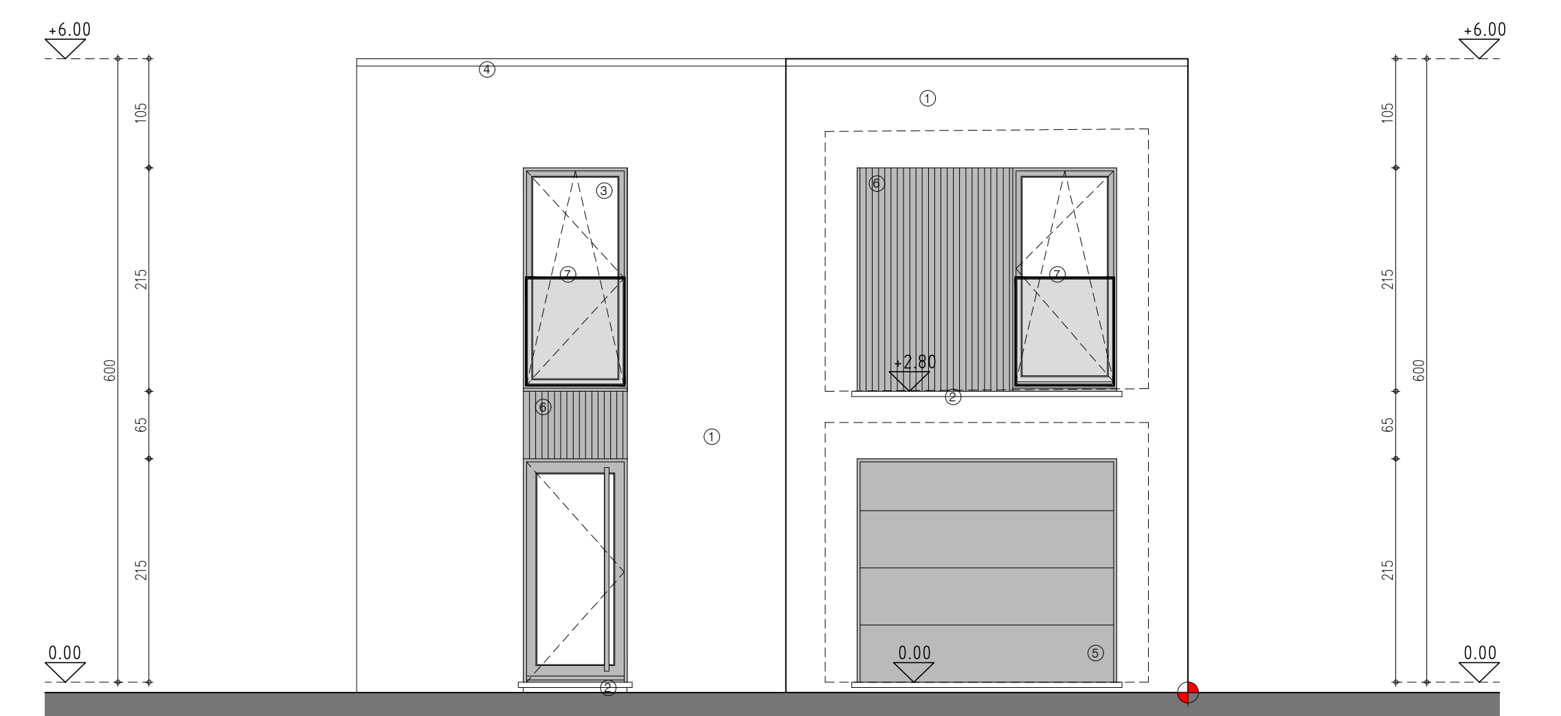
gevel zuid - voorgevel lot 77
