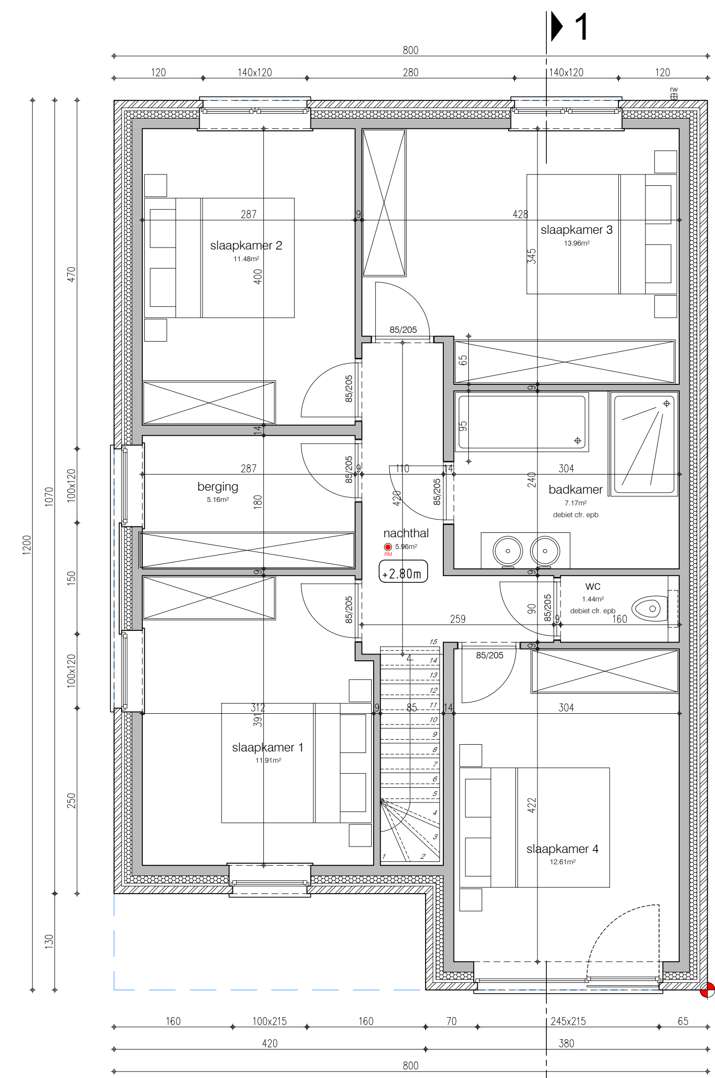
verdiepingsplan lot 77 90.54 m 2 bruto opp. 75.91 m 2 netto opp.
