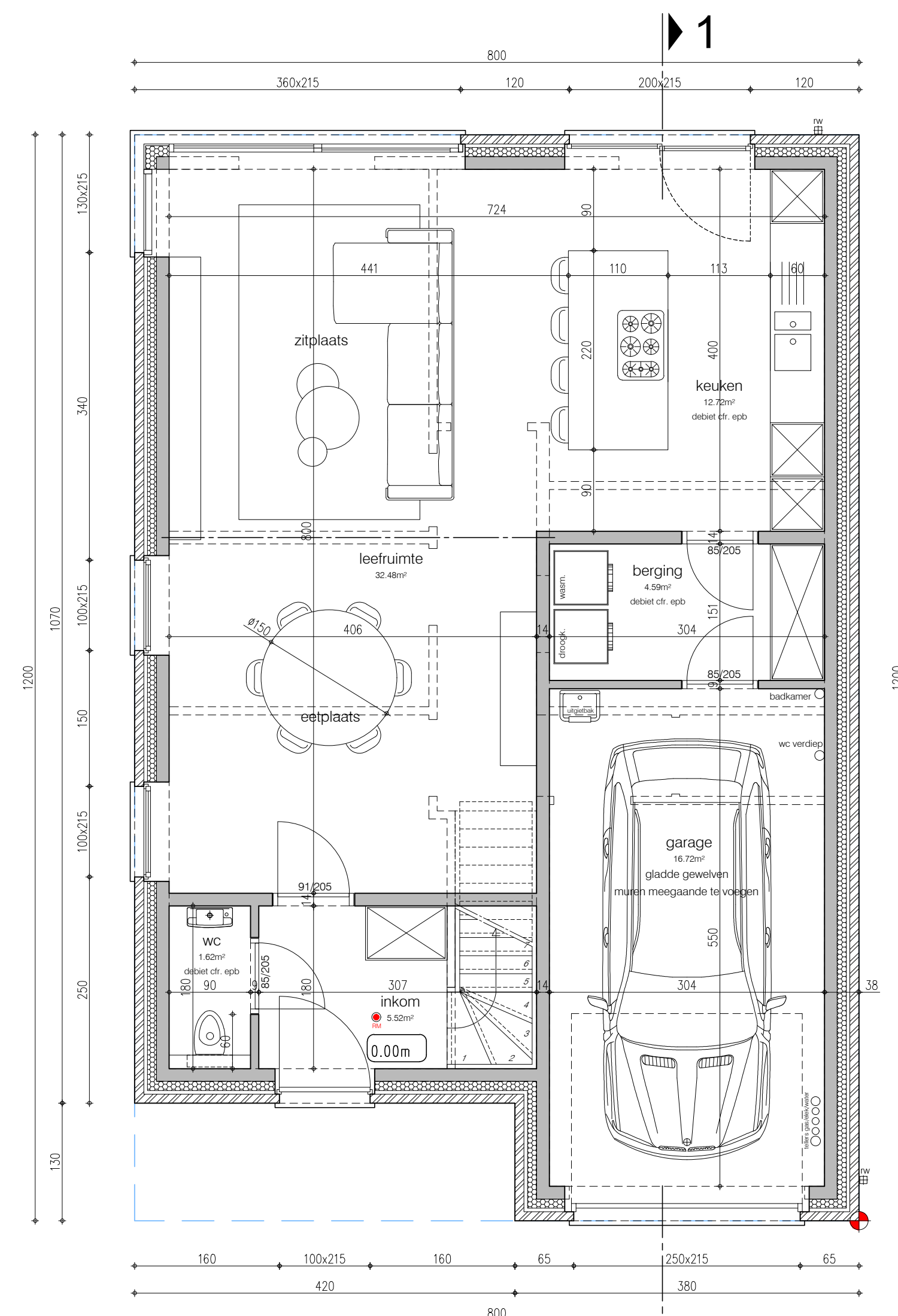
gelijkvloers lot 77 90.54 m 2 bruto opp. 75.91 m 2 netto opp.
