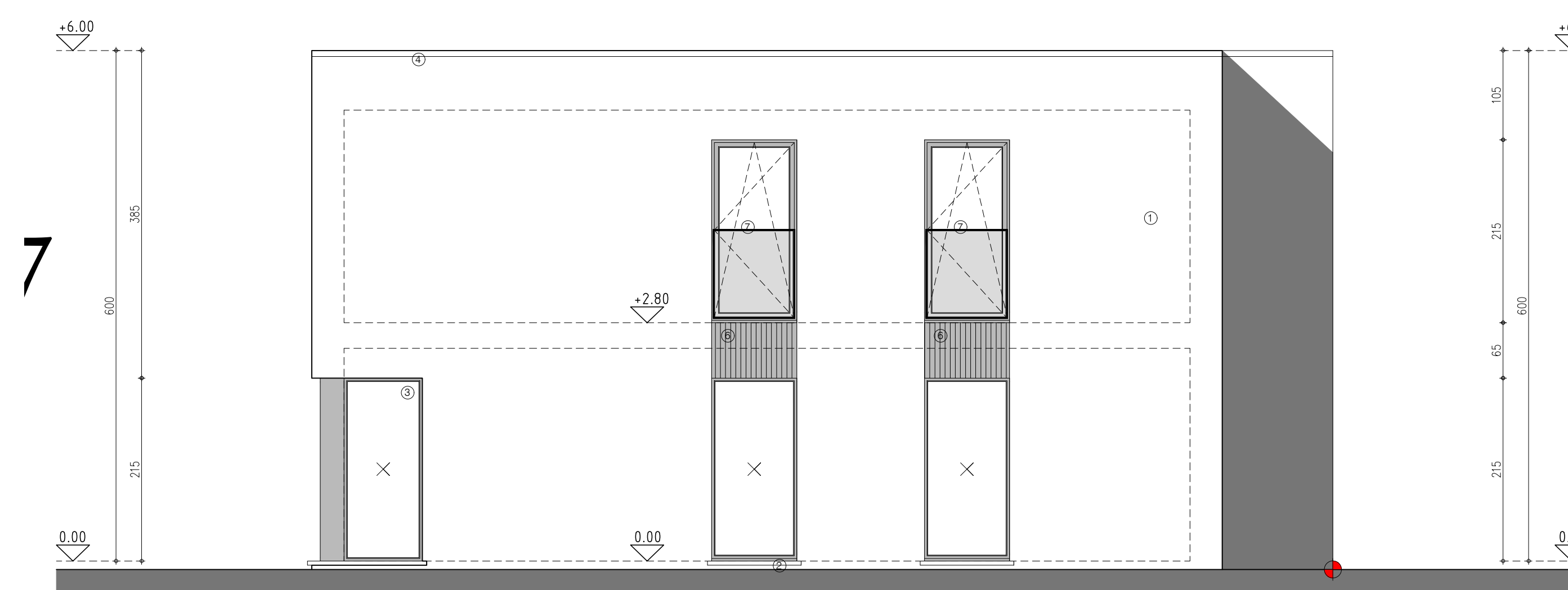
gevel west - linker zijgevel lot 77
